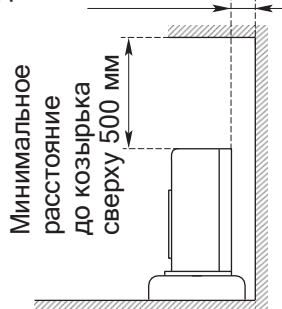
Размещение под козырьком Минимальное расстояние от задней стенки наружного блока до стены 100 мм
