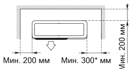
Размещение в нише со свободным выходом воздушного потока вперед
