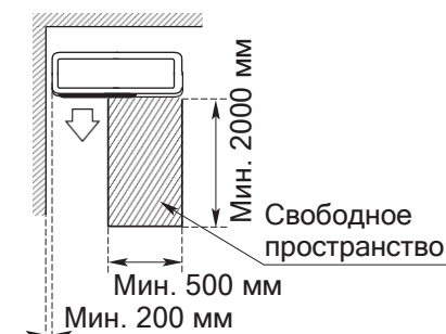
Рекомендуемое пространство для сервисного обслуживания
